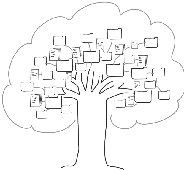
Abbildung 1.1: Gewachsener Ordnerbaum
