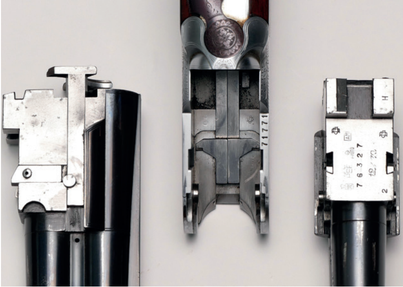
Abbildung 5: Verschlusskasten der Bockflinte (Mitte), die sogenannte Basküle – deutlich erkennbar sind die seitlichen und unteren Aussparungen, in die die Verriegelung des korrespondierenden Verschlussstückes der Laufpaare (links und rechts) eingreifen.
